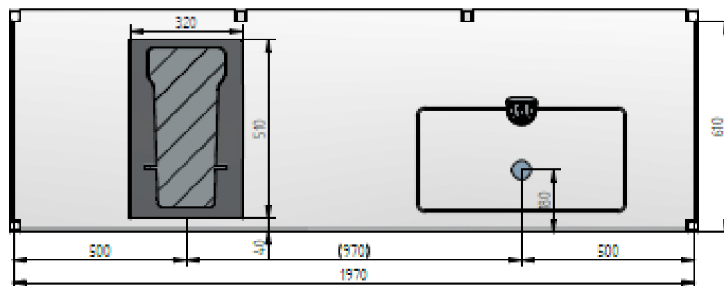
ŘEZ A-A Pracovní plocha
