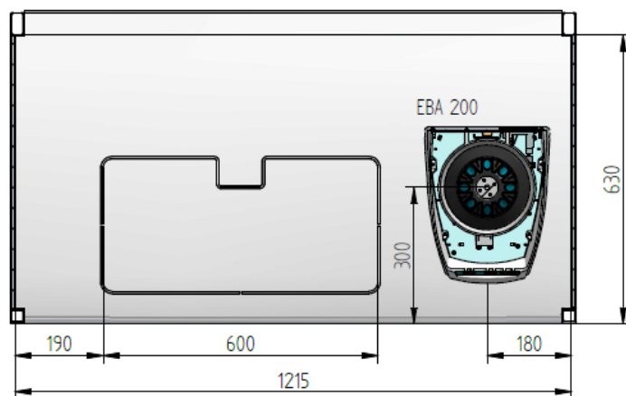
A-A Pracovní deska Work area
