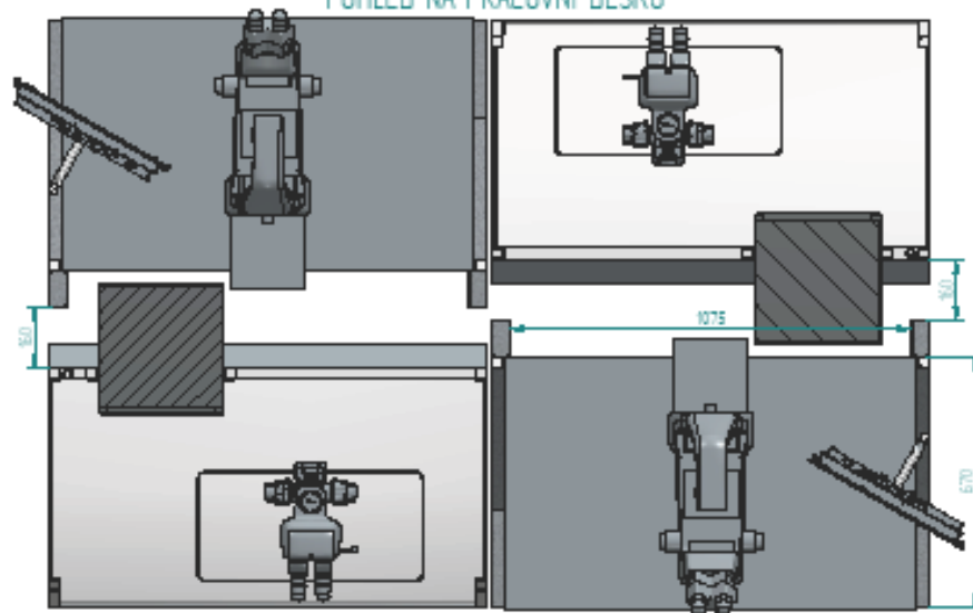
ŘEZ A-A POHLED NA PRACOVNÍ DESKU
