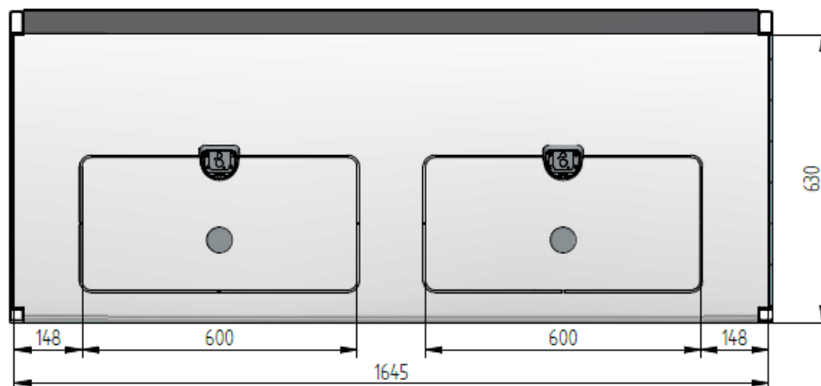
A-A Pracovní deska Work area
